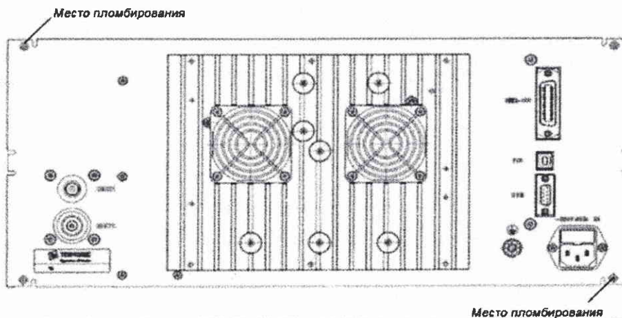
Рисунок 2 - Внешний вид калибратора (вид сзади)
